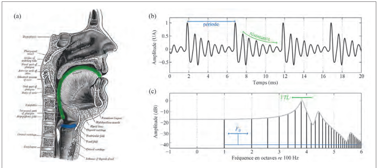
Fig. 1 : (a) Coupe sagittale de l'appareil vocal (d'après [36]). Les cordes vocales (la source) sont surlignées en bleu, et le tractus vocal (le filtre) est surligné en vert. (b) Forme d'onde de la voyelle /a/. La période des impulsions glottiques est mise en évidence par une flèche bleue. La durée de la résonance dans le tractus vocal est montrée par une flèche verte. (c) Spectre du même son. Les raies harmoniques sont montrées en noir, l'enveloppe spectrale est représentée en gris. La fréquence fondamentale ( F_0 ) est indiquée en bleu, et l'effet de la longueur du tractus vocal (VTL) est illustré en vert. Adapté de [6].
