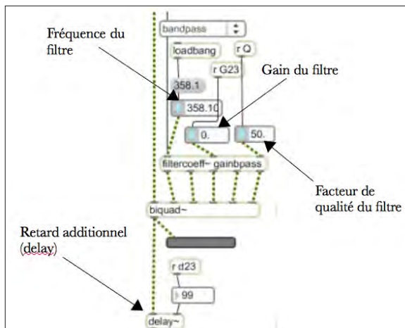
Fig. 5 : Filtre passe-bande dans Max/MSP utilisé pour le système de contrôle numérique
