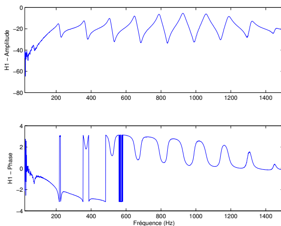
Fig. 3 : Fonction de transfert en boucle fermée du système avec contrôleur numérique (configuration sans contrôle actif)
