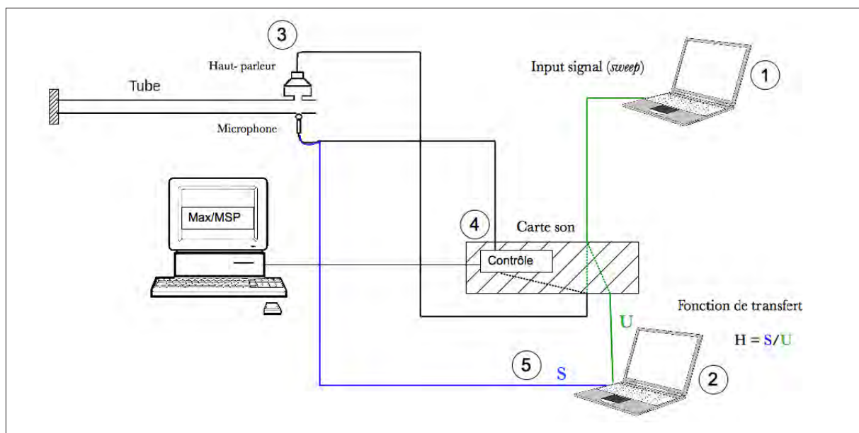
Fig. 2 : Dispositif expérimental pour la mesure de la fonction de transfert en boucle fermée du système
