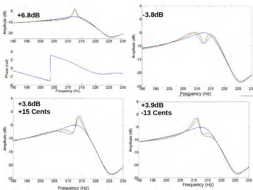
Fig. 6 : Différents contrôles appliqués à la deuxième résonance de l'instrument, FT mesurées sans contrôle (bleu), avec contrôle (rouge) et simulation de contrôle (vert). Les contrôles sont tous réalisés avec G = 1 et Q = 50 , et quatre phases ciblées différentes. Haut gauche : \phi_c = 0 . Haut droite : \phi_c = \pi . Bas gauche : \phi_c = \pi/2 , Bas droite : \phi_c = 3\pi/2
