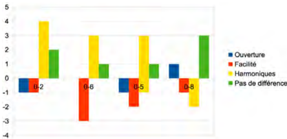
Fig. 11 : Effet de la phase pour les configurations avec un gain maximal, en comparaison avec la configuration sans contrôle. Configuration n°2 : \phi = 0 et G = 1,5 . Configuration n°6 : \phi = \pi/2 et G = 1 . Configuration n°5 : \phi = \pi et G = 3 . Configuration n°8 : 3\pi/2 et G = 1,5
