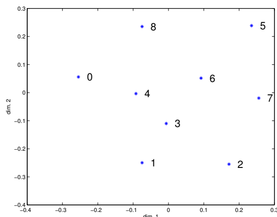
Fig. 8 : MDS INDSCAL de l'ensemble des matrices de dissemblances des 7 sujets. Les numéros des configurations sont identiques à ceux de la figure 7. Les paires les plus éloignées sont celles qui ont recueilli en moyenne les plus grands jugements de dissemblance de la part des musiciens.
