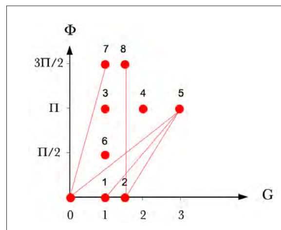
Fig. 7 : Espace des paramètres pour les configurations testées dans notre expérience. En abscisse, le gain des filtres, en ordonnée le déphasage imposé. Les paires de configurations reliées par des traits rouges sont les paires ayant recueilli en moyenne, par la suite, les plus grands jugements de dissemblance (voir Chapitre Consensus des musiciens page 15).
