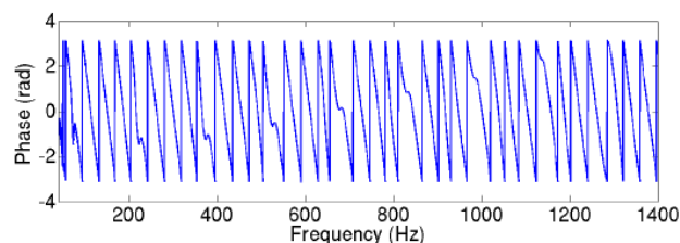
Fig. 4 : Phase en boucle ouverte de la fonction de transfert du système
