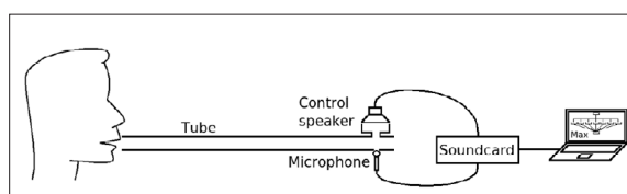
Fig. 1 : Schéma simplifié du système de contrôle numérique monté sur le système tube+anche
