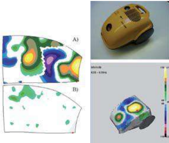
Fig. 2: Left: Measurements on a car window during wind tunnel tests. A: with mirror, B: without mirror, intensity at 125 Hz 1/3rd octave. Right: Vacuum cleaner, intensity 630 Hz 1/3rd octave. Gauche : Mesures sur une fenêtre de voiture pendant des tests en soufflerie. A : avec un rétroviseur, B : sans rétroviseur, intensité au 1/3 d'octave 125 Hz. Droite : Aspirateur, intensité au 1/3 d'octave 630 Hz.
