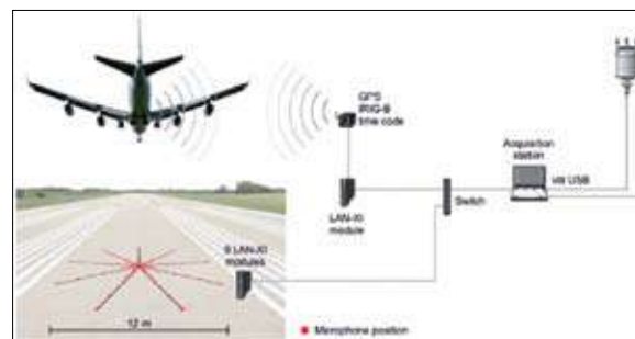
Fig. 6 : Typical system for measurement and data acquisition for Noise Source Identification during flyover of passenger aircraft using Moving Source Beamforming Système caractéristique d'acquisition des mesures et des données pour NSI lors de l'atterrissage d'un avion de ligne en utilisant la méthode des faisceaux pour sources mouvantes
