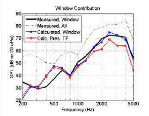
Fig. 3 : Pressure contribution at the driver's ear position of a flat loudspeaker attached on a window of a car cabin. The measured true contribution corresponds to solid black curve, the calculated contribution correspond to solid blue curve. For the red curve only the operational particle velocity is used. Contribution de la pression d'un haut-parleur plat fixé au niveau de l'oreille du conducteur, sur la fenêtre de l'habitacle d'une voiture. La contribution véritablement mesurée correspond à la courbe noire, la contribution calculée correspond à la courbe bleue. Pour la courbe rouge, uniquement la vitesse des particules opérationnelles est utilisée.
