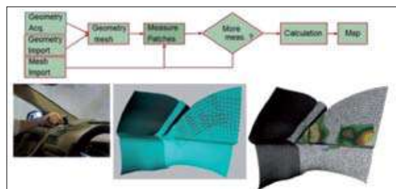
Fig. 1: Conformal mapping workflow : Import or acquisition of the geometry, mesh generation, patch measurements, calculations and displays Déroulement du travail de cartographie : importation ou acquisition de la géométrie, génération du maillage, mesures de correction, calculs et affichage
