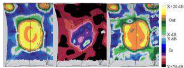
Fig. 4 : SONAH calculations. Left: Transmission loss noise without emission from loudspeakers (reference). Middle: Transmission loss with emission from loudspeakers. Right: Transmission loss with emission from loudspeakers, but with Entering Intensity processing applied. Exemples de calculs avec SONAH. Gauche : perte de transmission du son d'un haut-parleur sans émission (référence). Au centre : perte de transmission du son d'un haut-parleur en fonctionnement. Droite : perte de transmission d'un haut-parleur en fonctionnement mais avec l'application d'un traitement d'intensité entrante.
