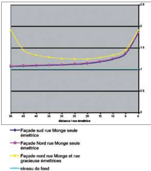
Fig. 5 : Niveau de pollution le long des façades Nord et Sud de la place Monge par rapport à un niveau de référence (ici 1 000 \mu\text{g}/\text{m}^3 de CO)
