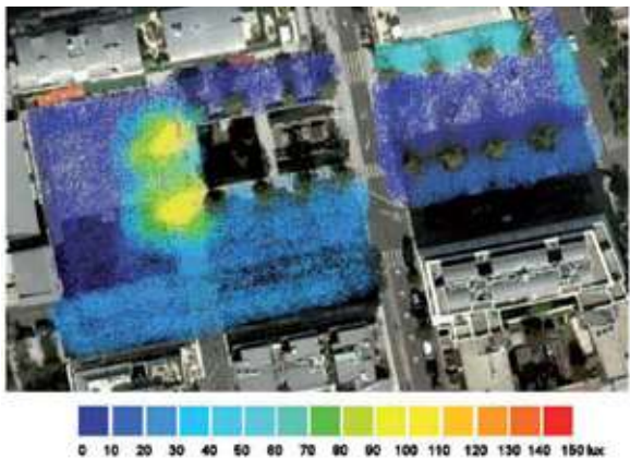
Fig. 2 : Cartographie des éclairages horizontaux mesurés à 1m de hauteur Grand'place, Boulogne Billancourt
