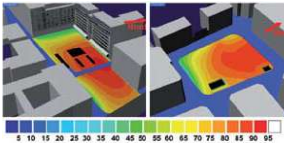
Fig. 4 : Pourcentage d'ensoleillement en lux. Heure/référence en site dégagé (à gauche : Grand'place, à droite : place Monge)
