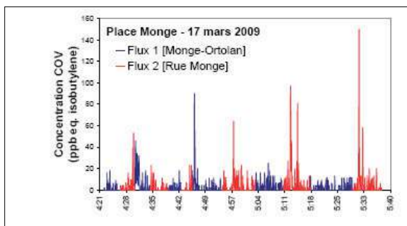
Fig. 6 : Concentration de COV mesurée place Monge en déplacement selon les trajets piétonniers
