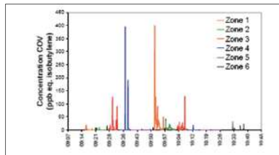
Fig. 7 : Concentration de COV mesurée Grand'place en déplacement selon six zones caractéristiques
