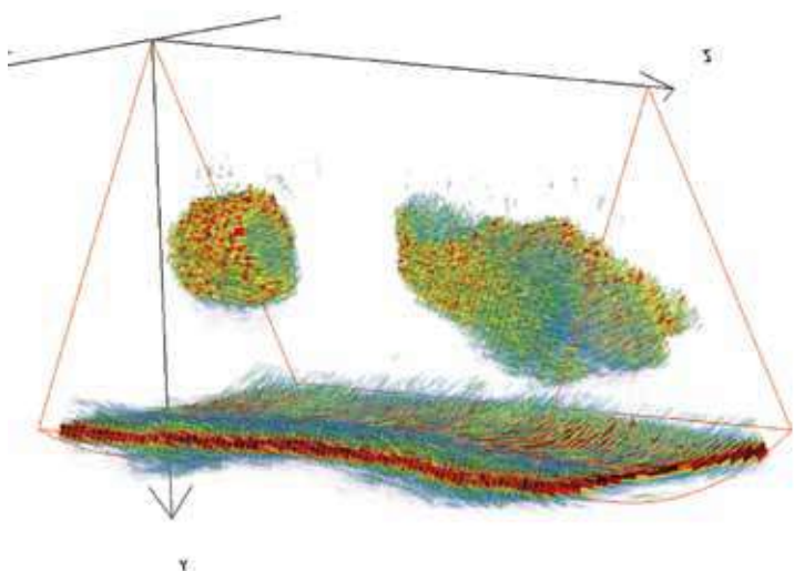
Fig. 2 : Représentation 3D d'échos de bancs de poissons et du fond obtenus avec le sondeur multifaisceau du N.O. Thalassa
